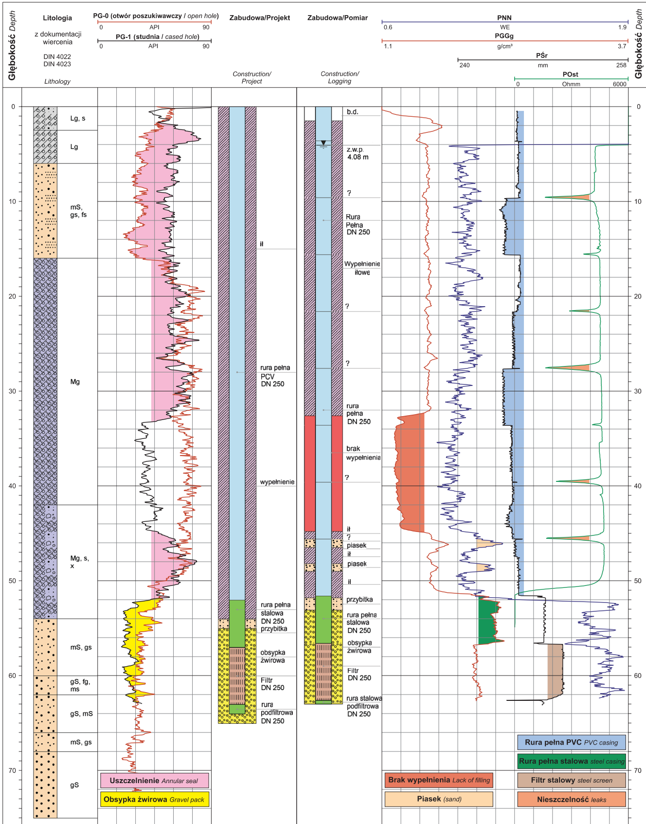
Fig. 1. Kontrola studni z udokumentowanym brakiem wypełnienia przestrzeni pierścieniowej
